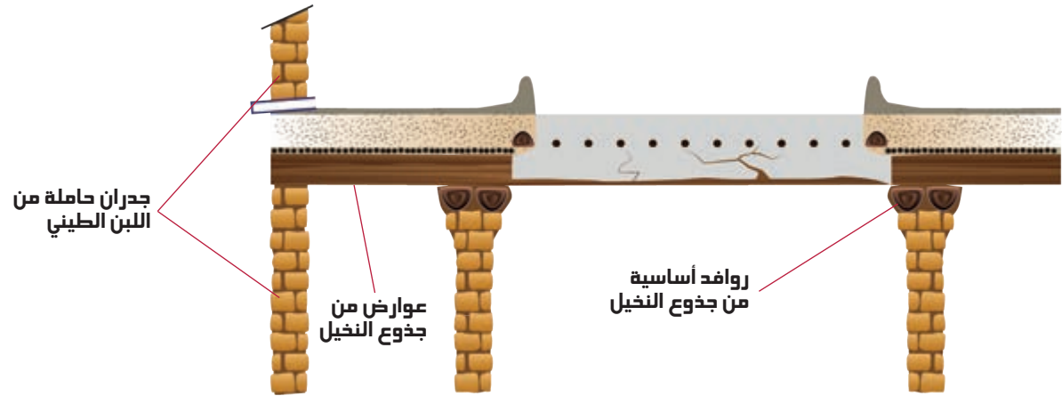
مقطع على مستوى وسط الدار
