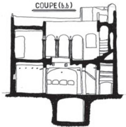
مقطع B-B
