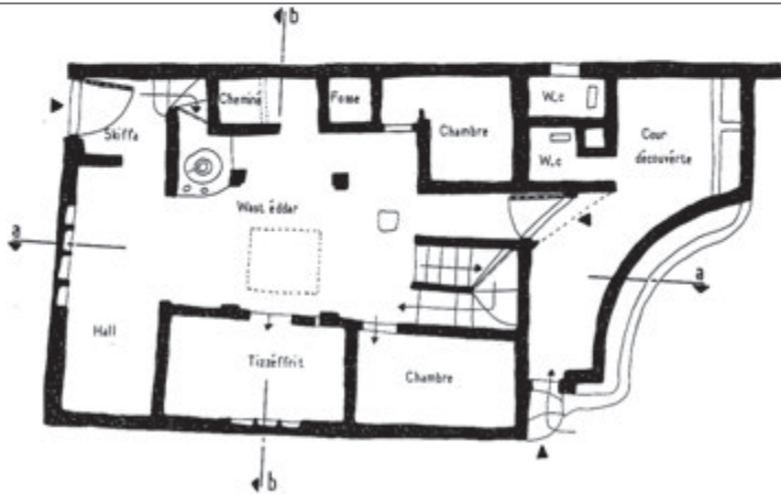
مخطط الطابق الأرضي
